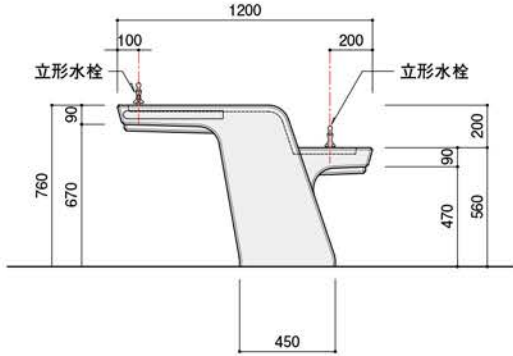
[立面図]
