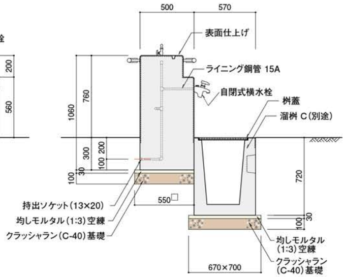
[施工断面図]
