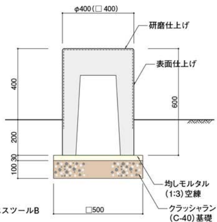
[施工断面図(固定式)]
